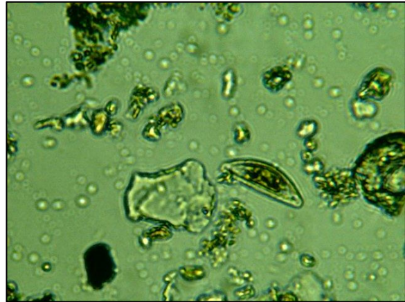
Fotografía 10. Cymbella sp. Clase Bacillariophyceae
