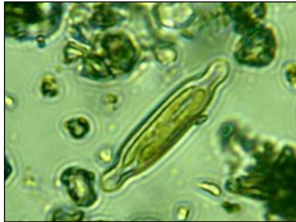
Fotografía 16. Stauroneis sp. Clase Bacillariophyceae
