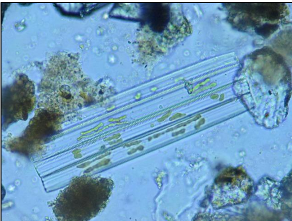
Fotografía 7. Fragilaria sp. Clase Fragilariophyceae
