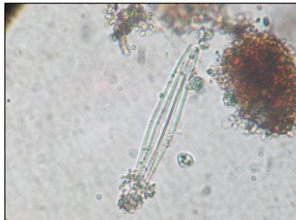
Fotografía 12. Frustulia sp. Clase Bacillariophyceae
