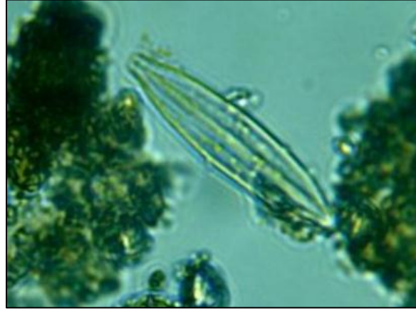
Fotografía 14. Navicula sp. Clase Bacillariophyceae
