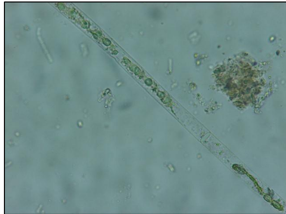
Fotografía 4. Mougeotia sp. Clase Zygnematophyceae
