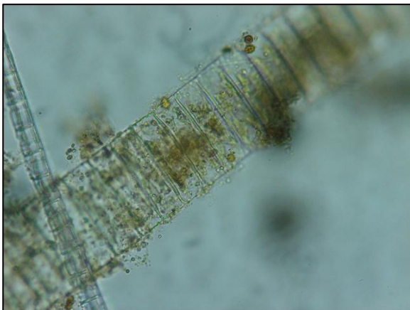
Fotografía 11. Eunotia sp. Clase Bacillariophyceae
