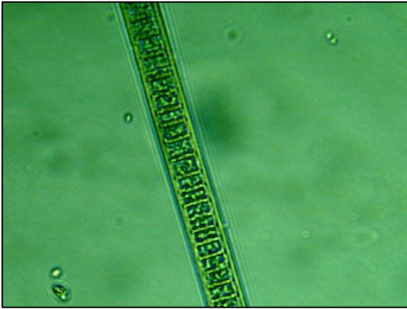
Fotografía 21. Oscillatoria sp. Clase Cyanophyceae
